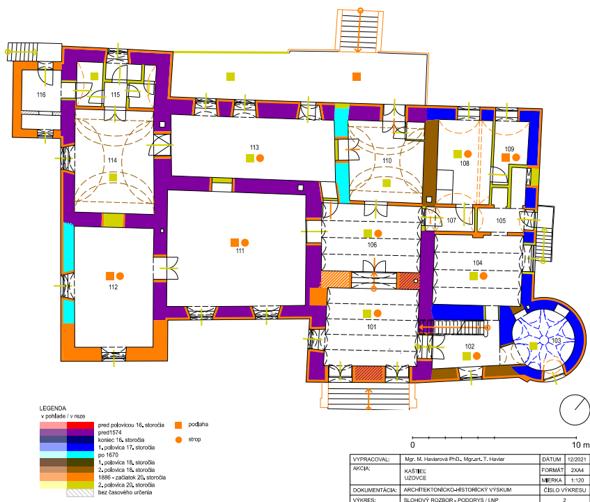
Kaštieľ v Uzovciach, analýza stavebného vývoja suterénu a prízemí kaštieľa na základe architektonicko-historického výskumu
