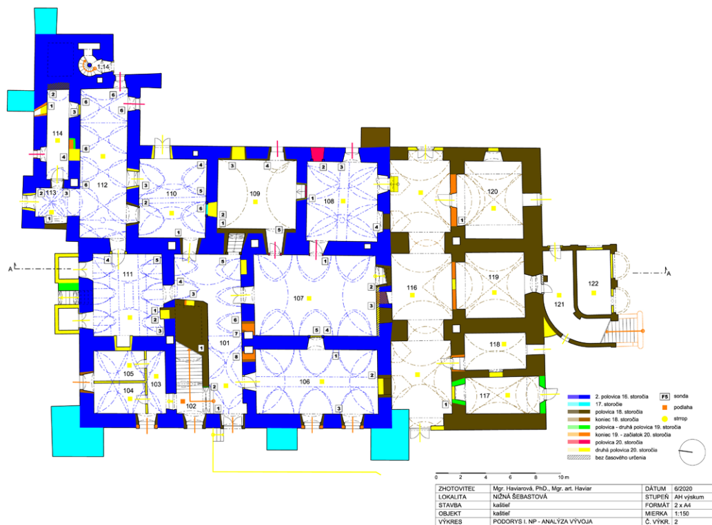
Kaštieľ v Prešove - Nižnej Šebastovej, analýza stavebného vývoja prízemia kaštiľa na základe architektonicko-historického výskumu
