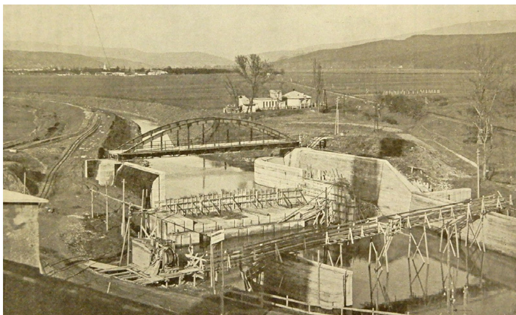
Obr. 4: Pohled na staveniště vodní elektrárny v Užhorodě a na přívodní kanál z března 1937.
