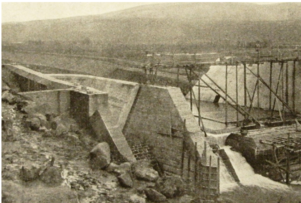
Obr. 3: Pohled na část staveniště vodní elektrárny mezi Nevickým a Onokovcami s přívodním kanálem z března 1937. MACH, Vladimír. Využití vodních sil na Podkarpatské Rusi. In Ant. Kubart (ed.): Vodohospodářské otázky Podkarpatské Rusi. Meliorační svaz pro Podkarpatskou Rus v Užhorodě. 1927 – 1937. Užhorod : Meliorační svaz pro Podkarpatskou Rus, 1937, s. 54.
