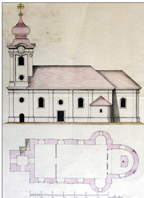
Obrázok 16 Trojpriestorový typizovaný projekt pre gréckokatolícke chrámy z roku 1797 (Zdroj: Державний архів Закарпатської області Берегове, Государственный архив Закарпатской области, фонд № 151, опись № 5, Един. Хран. № 1670/1)
