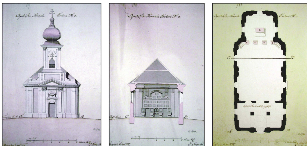
Obrázok 6 Tretia verzia typizovaného projektu Vavrince Landera pre gréckokatolícke chrámy z roku 1779 (Zdroj: Magyar Országos Levéltár Budapest, Tervtár, spis. š. T.1., fasc. č. 6, inv. č. 590, sign. 9 – 11)
