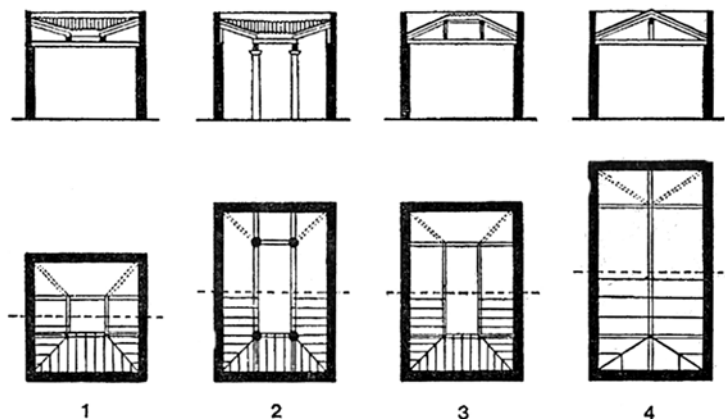
Typy átria podľa Vitruvia (rez a pôdorys): 1. toskánske, 2. štvorstĺpové, 3. bezokapové, 4. úplne prekryté 20
