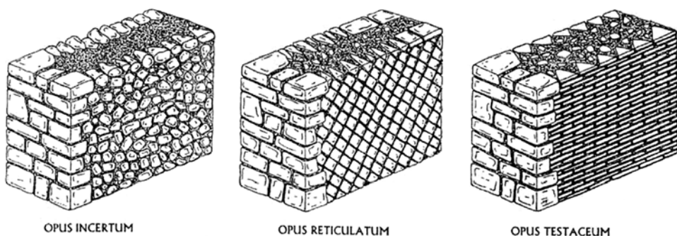
Tri hlavné typy rímskeho betónového muriva triedeného podľa typu vonkajšieho obkladu 8
