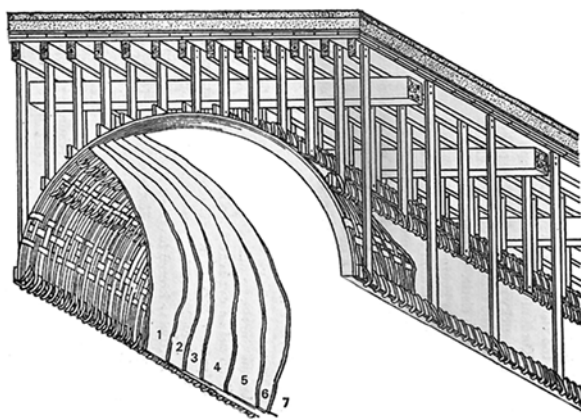
Tzv. falošná klenba zhotovená z drevenej konštrukcie, na ktorej je nanosených až sedem vrstiev omietky, podľa Vitruvia 12
