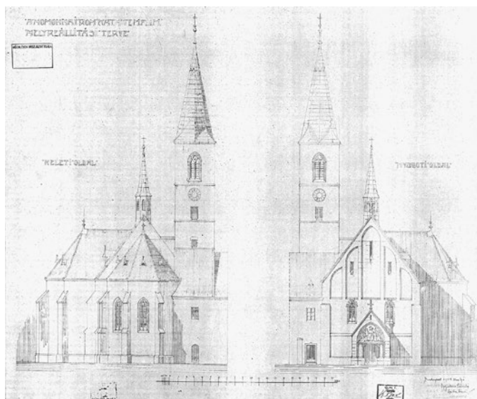
Obr. 8. Projekt Lászla Gyalusa na neogotickú prestavbu kostola z novembra 1905 – pohľad západný a východný.
